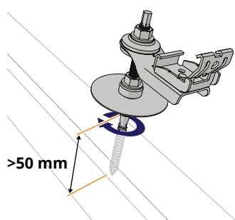
Bitumen or EPDM roofing
