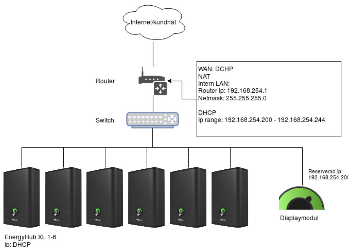
ILLUSTRATION 1: NÄTVERKSDIAGRAM
